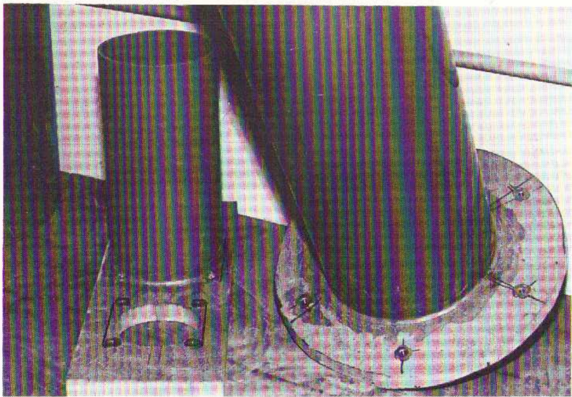
De bodemflens en de frontplaat (met aangeliijmde pijpen) De inslagmoeren zijn duidelijk te zien.
